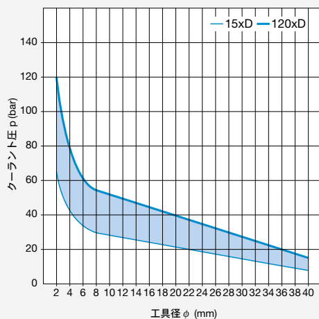
ZB 80 工具の長さによる推奨油圧
