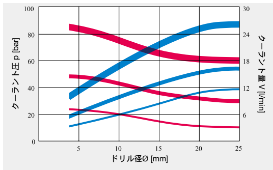
図4: AlSi合金加工での直溝RT150GGドリルに必要なクーラントの圧力と量
