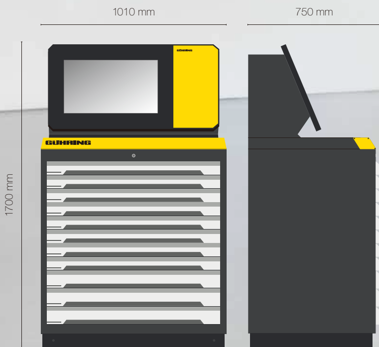
TM 326 ベーシックユニット・正面と側面
