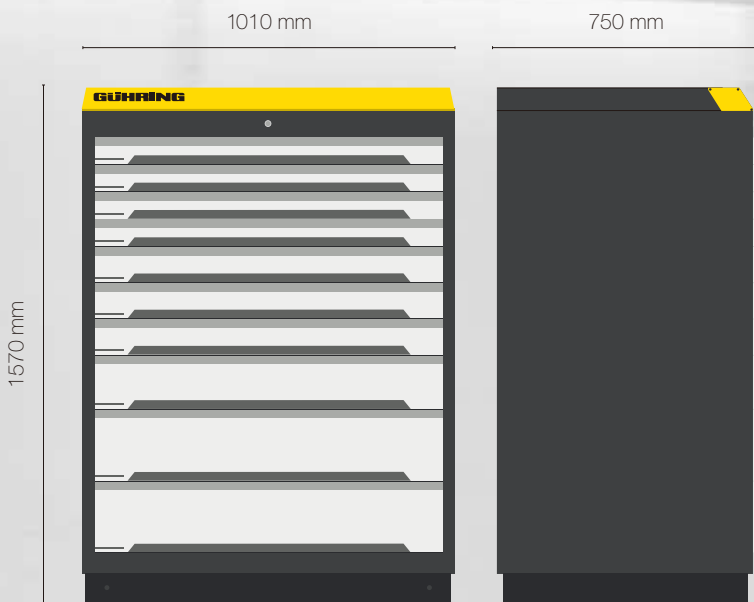
TM 326 拡張ユニット・正面と側面 (高さ: 1570 mm)
