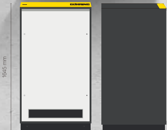
TM 426 スパイラルシステム 正面と側面
