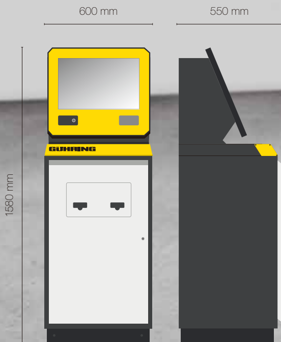
TM 426 制御端末の正面と側面
