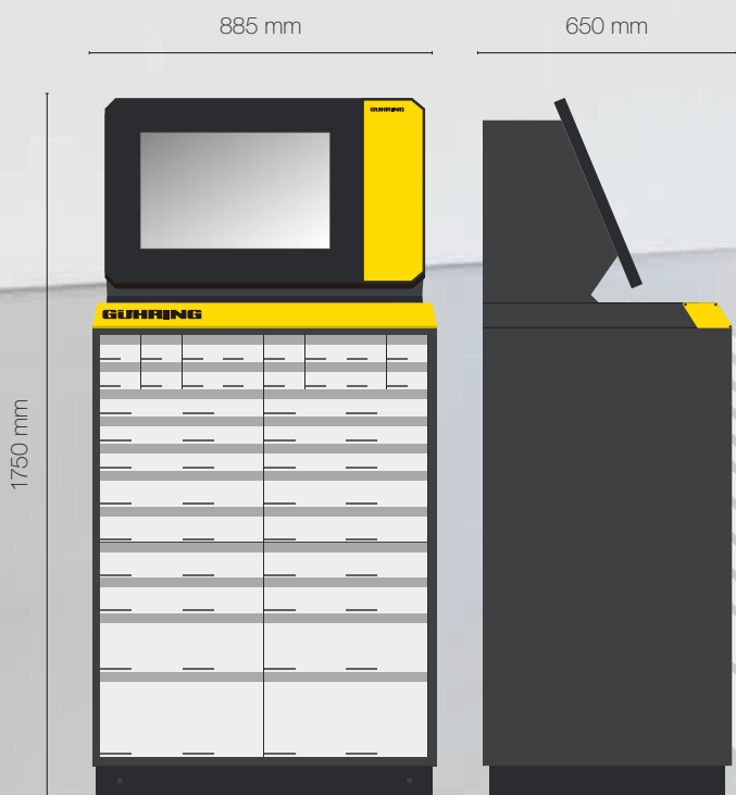
TM 526 ベーシックユニット・正面と側面
